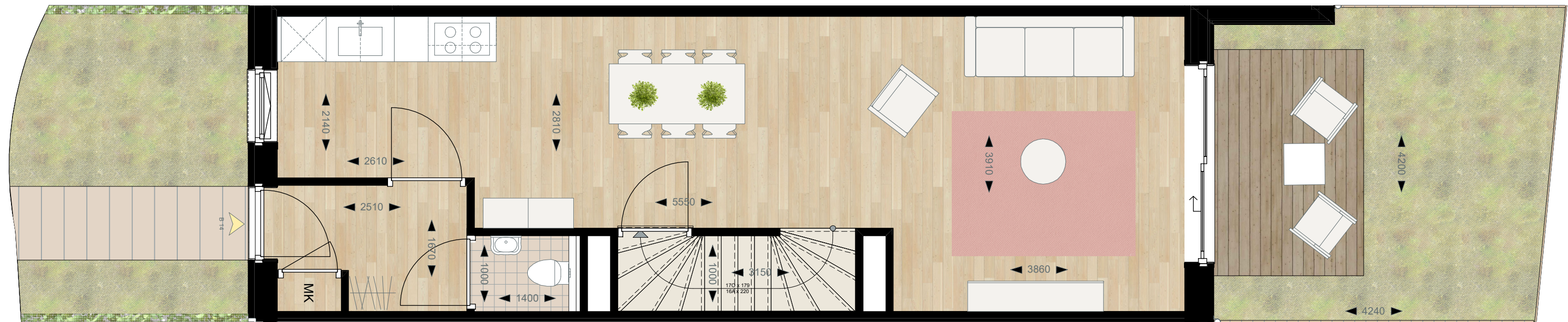
begane grond - schaal 1:50
