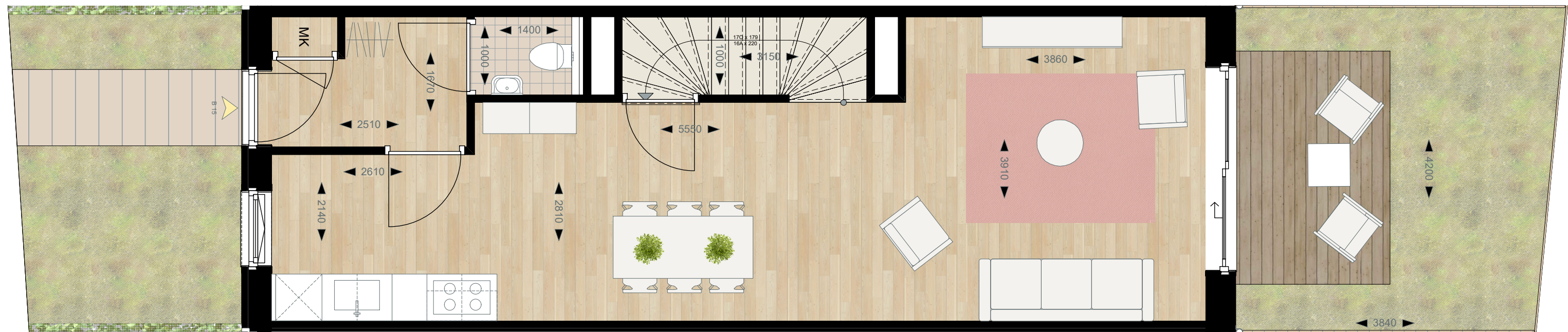
begane grond - schaal 1:50
