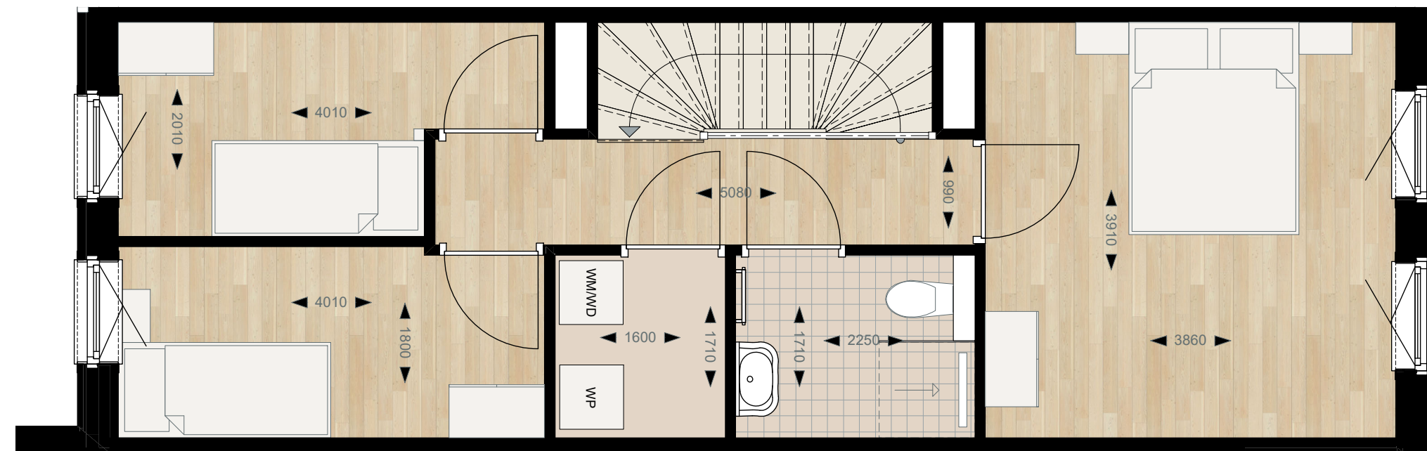
eerste verdieping - schaal 1:50
